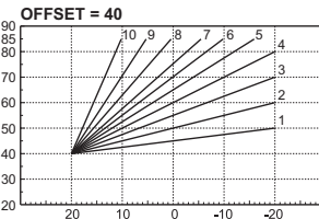
slika 15- Primjer paralelnog pomaka krivulja kompenzacije
