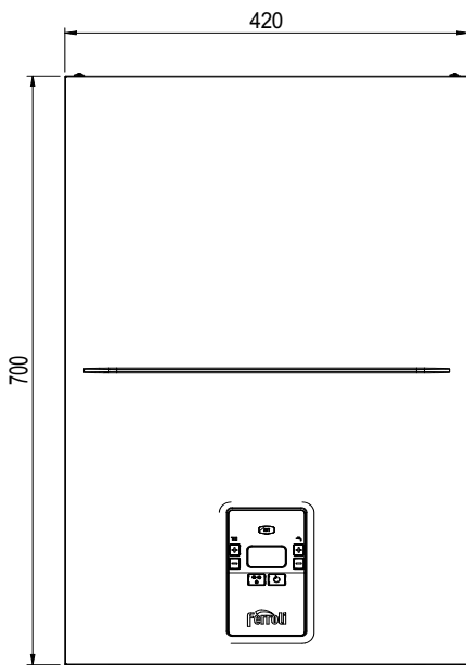
slika 32- Pogled sprijeda
